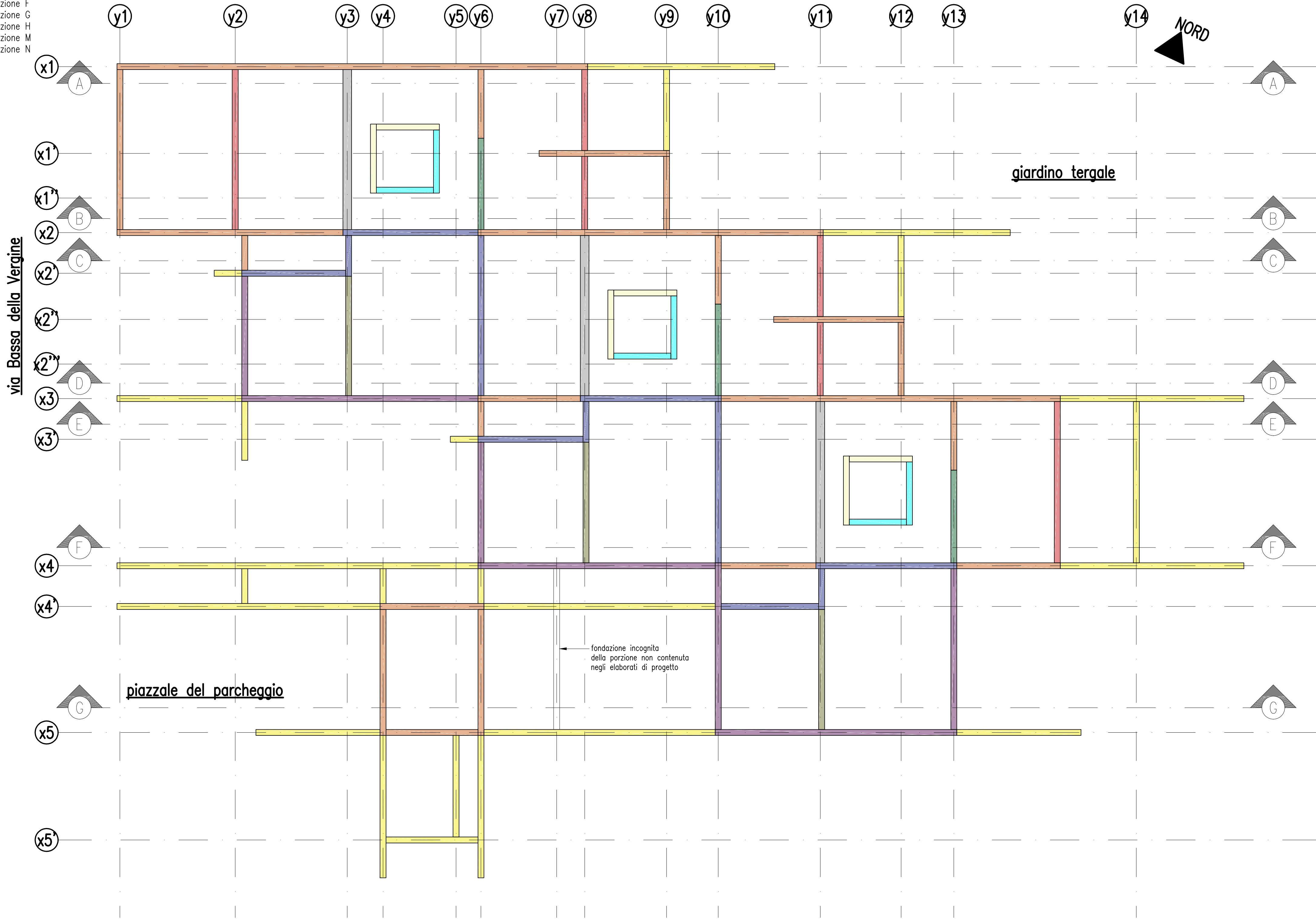
PIANTA DELLE FONDAZIONI – scala 1:100
