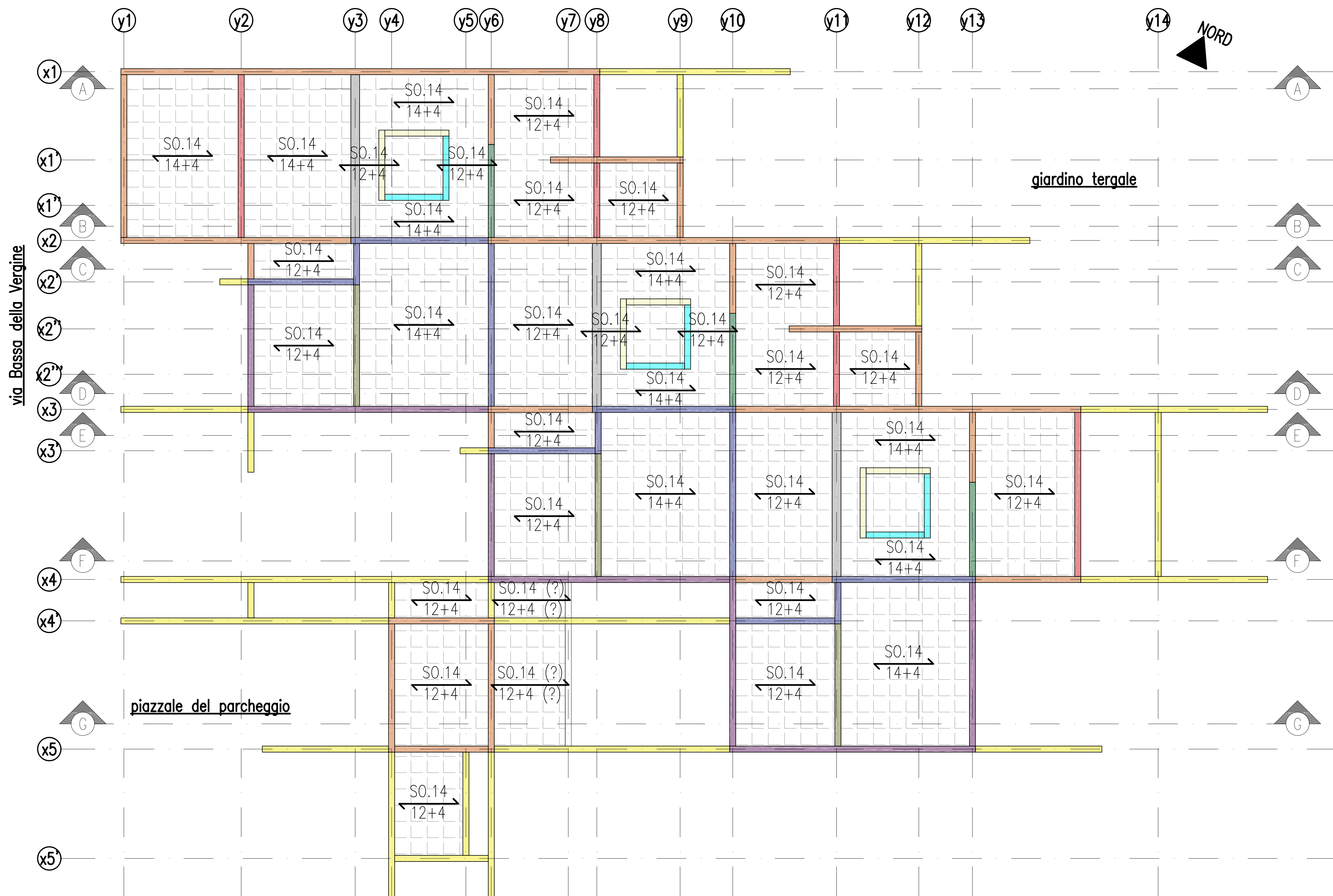
PIANTA DEI SOLAI DEL PIANO TERRA – scala 1:100
