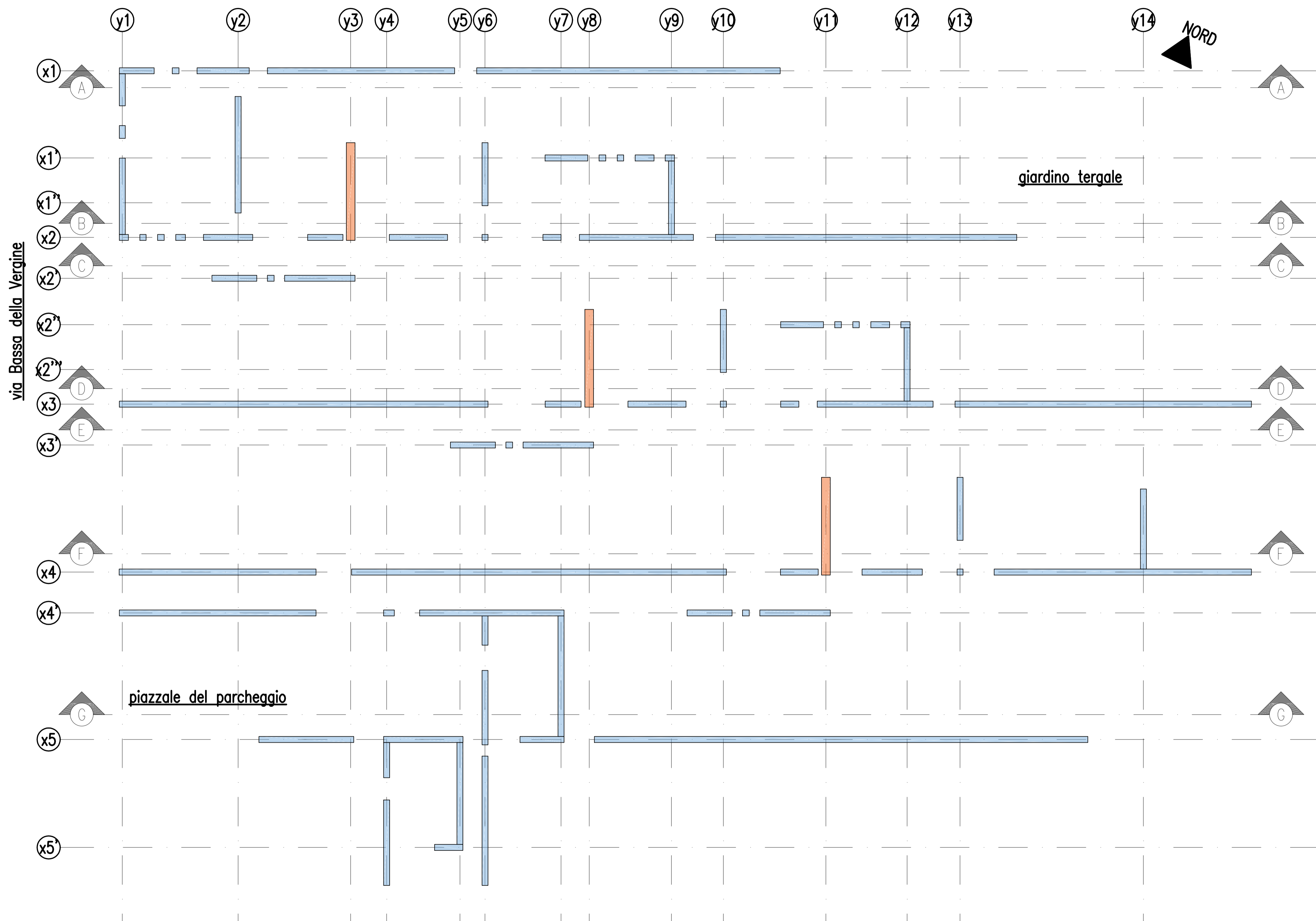
PIANTA DEI MURI DEL PIANO TERRA – scala 1:100
