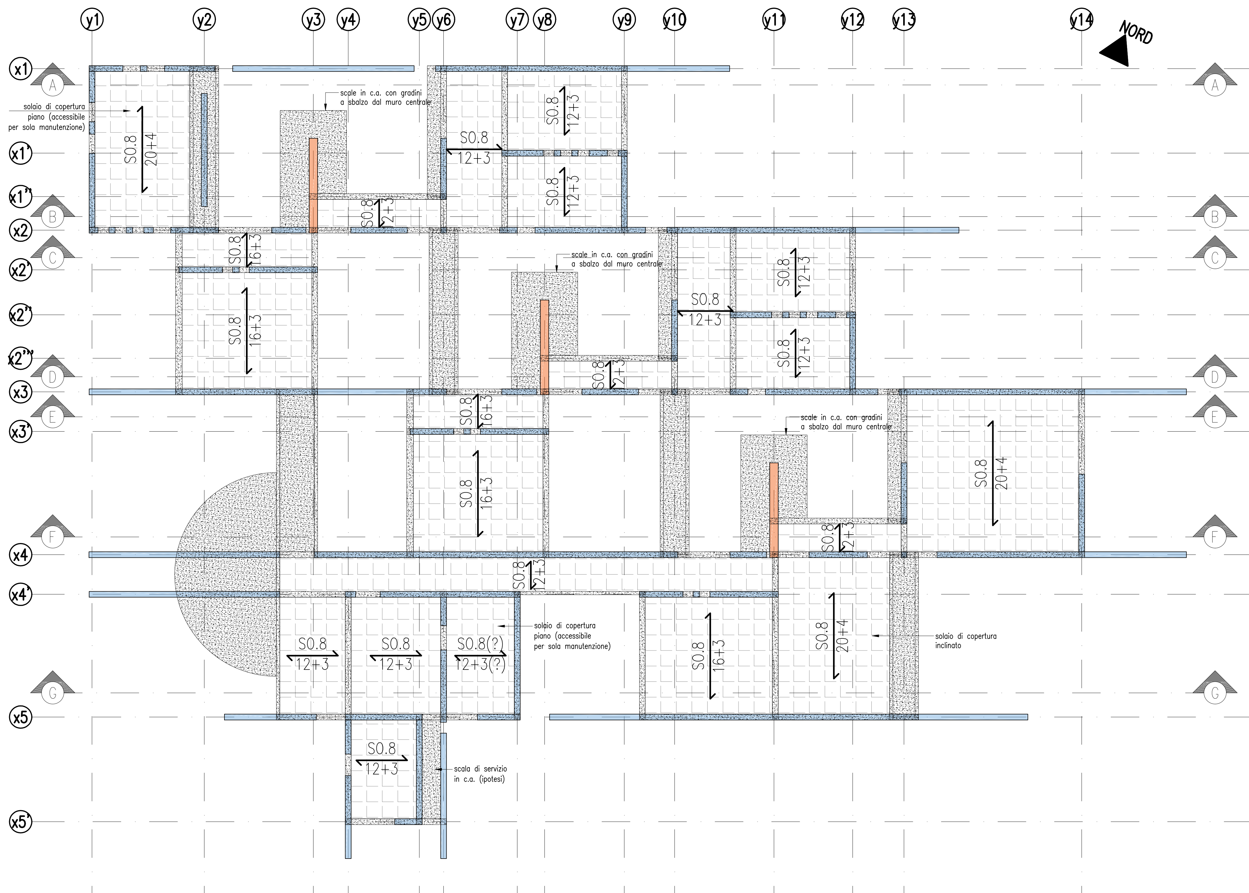
PIANTA DEI SOLAI DEL PIANO PRIMO – scala 1:100
