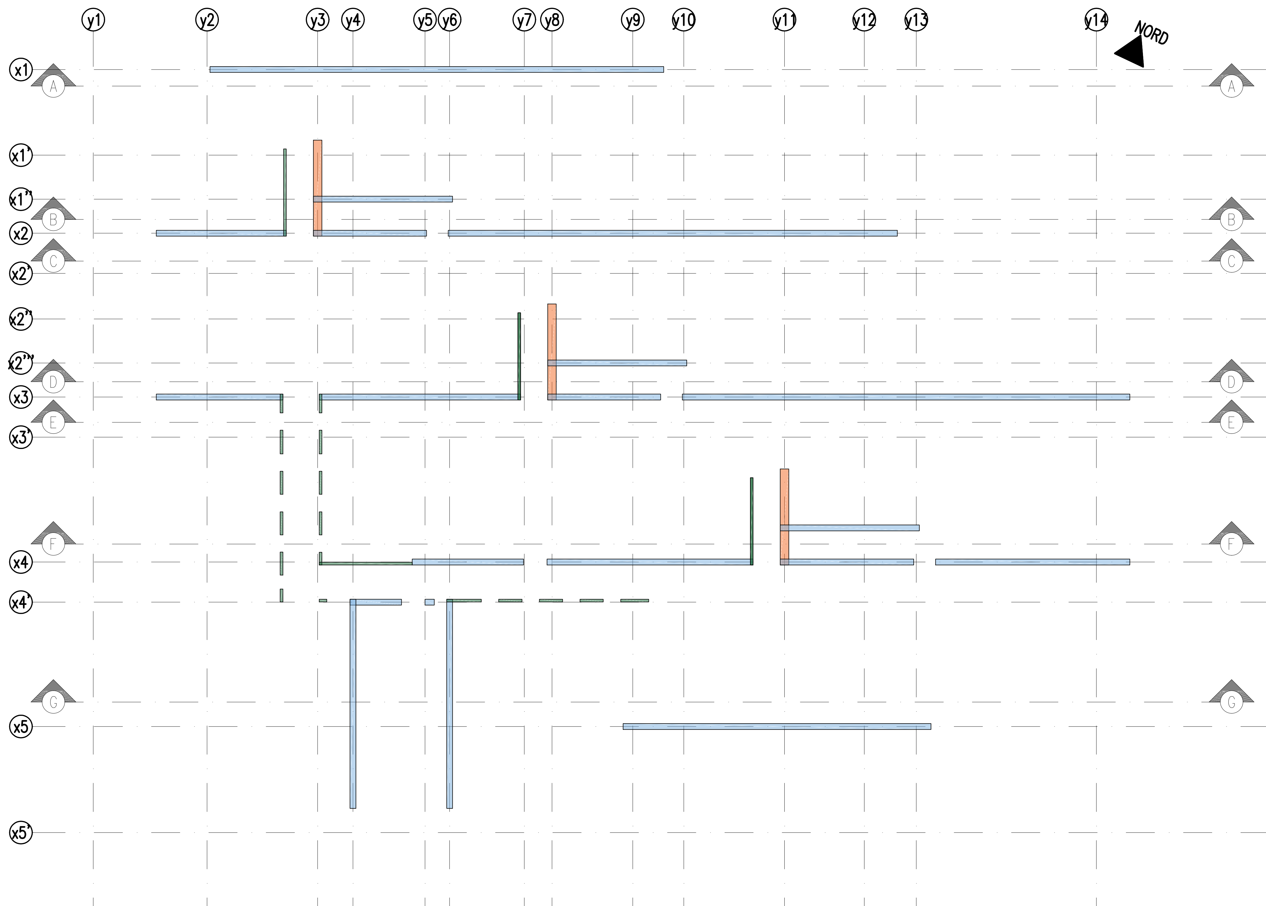
PIANTA DEI MURI DEL PIANO PRIMO – scala 1:100
