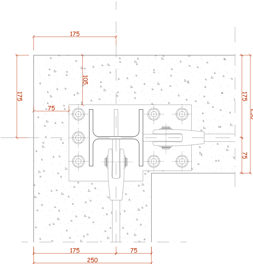
PLANIMETRIA NODO MONTANTE-FOSSA
