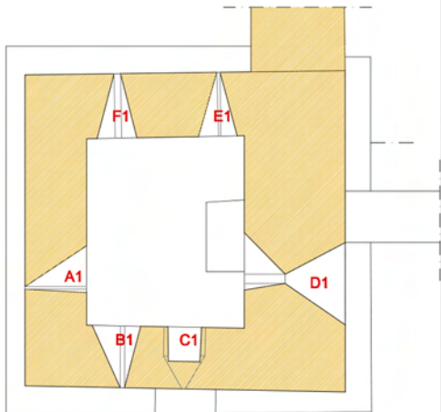
PIANTA LIVELLO +7.60
