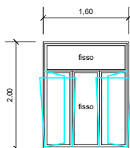
INFISSI TIPO "D" n° 5
