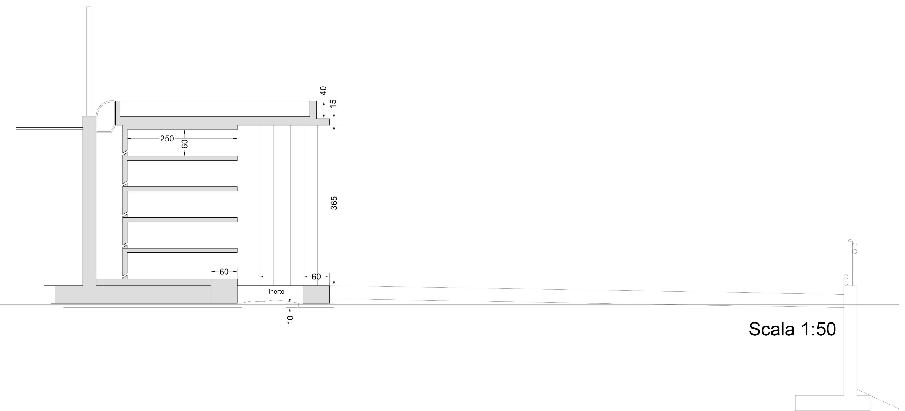
Sezione A-A
