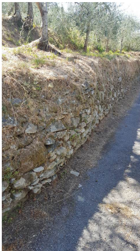
Figura 12 – Tratto di muro spanciato dove effettuare operazioni di scuci-cuci
