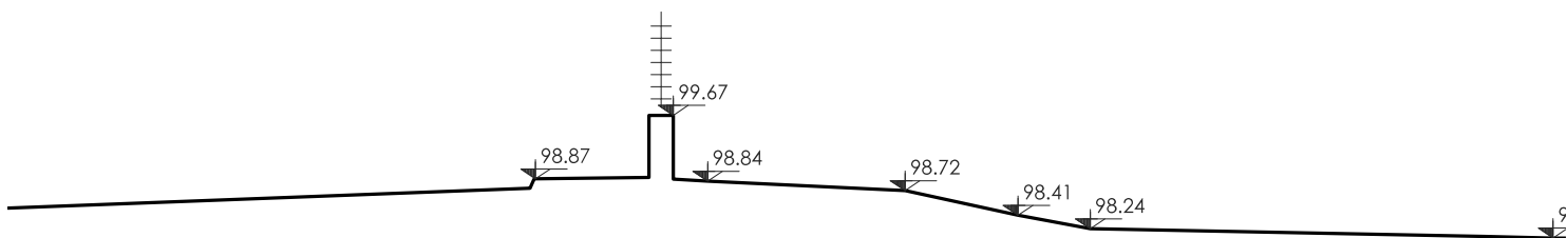
SEZIONE TERRITORIALE 3-3
