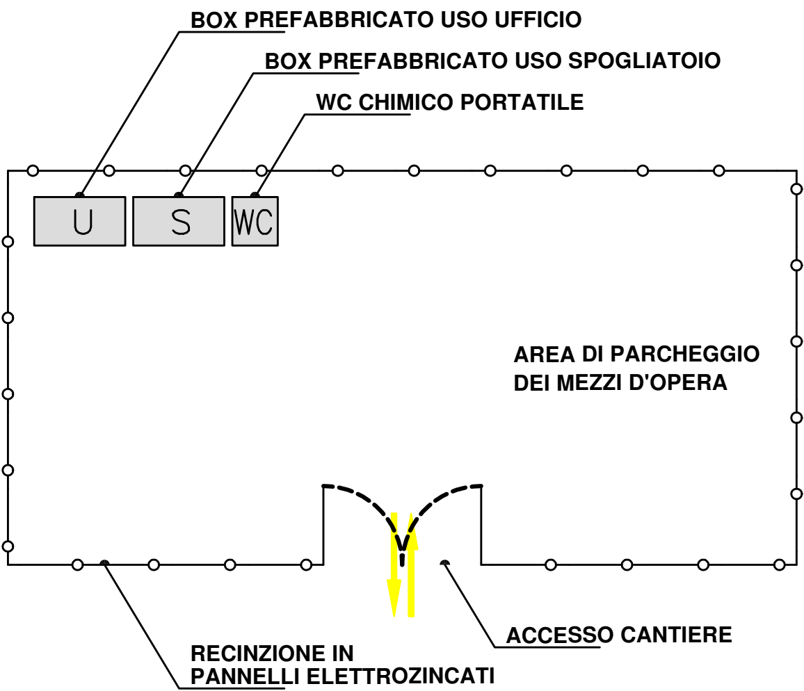
LAYOUT CAMPO BASE (SCHEMA TIPO):
