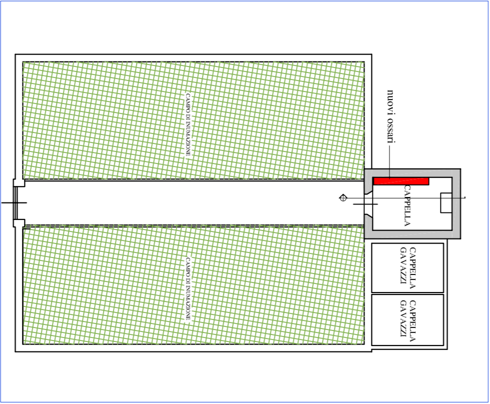
PLANIMETRIA GENERALE - scala 1:200
