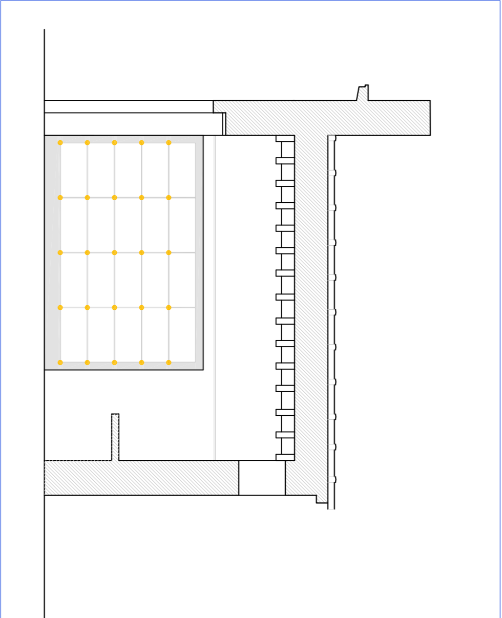
SEZIONE STATO MODIFICATO -scala 1:50
