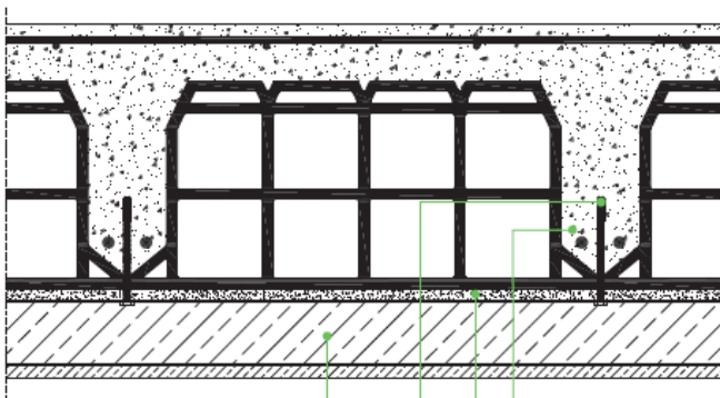
sezione trasversale ai travetti
