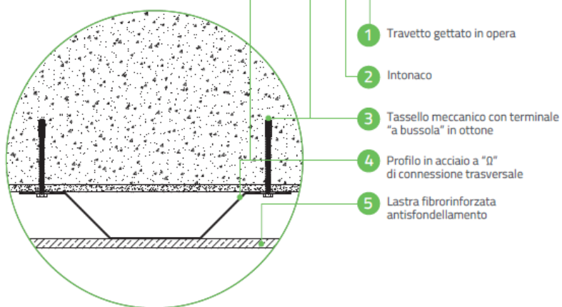
sezione longitudinale ai travetti
