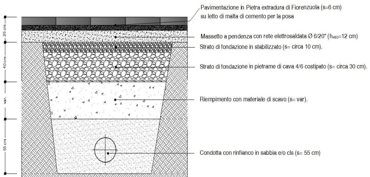
Fig. 3 - Sezione Riempimento Tipo sulla condotta Pluviale
