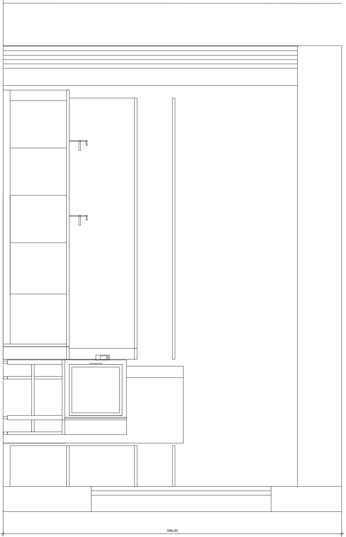
SEZIONE - PROSPETTO PARETE ATTREZZATA APERTA 1:25
