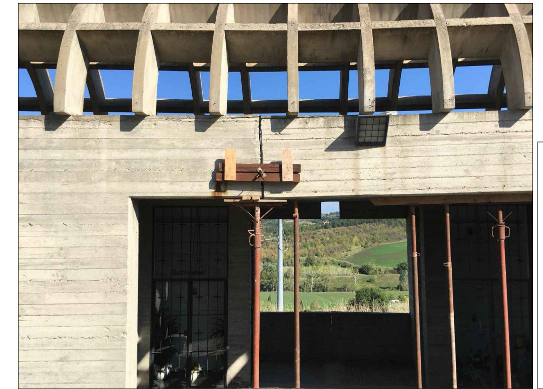
Lesione muro corridoio loculi
