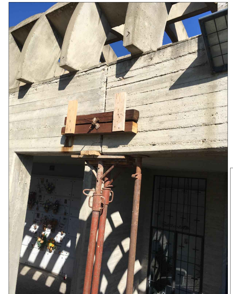
Lesione muro corridoio loculi
