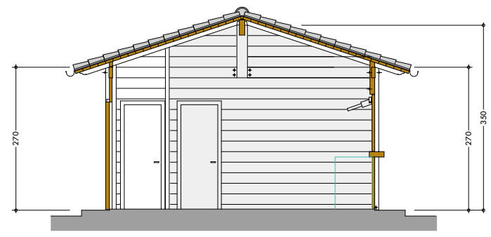
SEZIONE A-A
