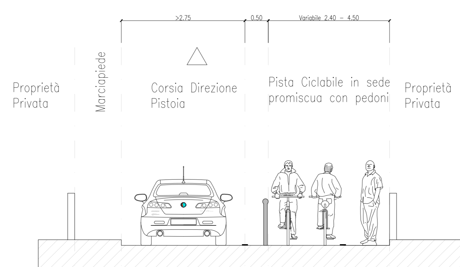
Stato di Progetto via Aiaccia intersezione Via Mastrigalla scala 1:50
