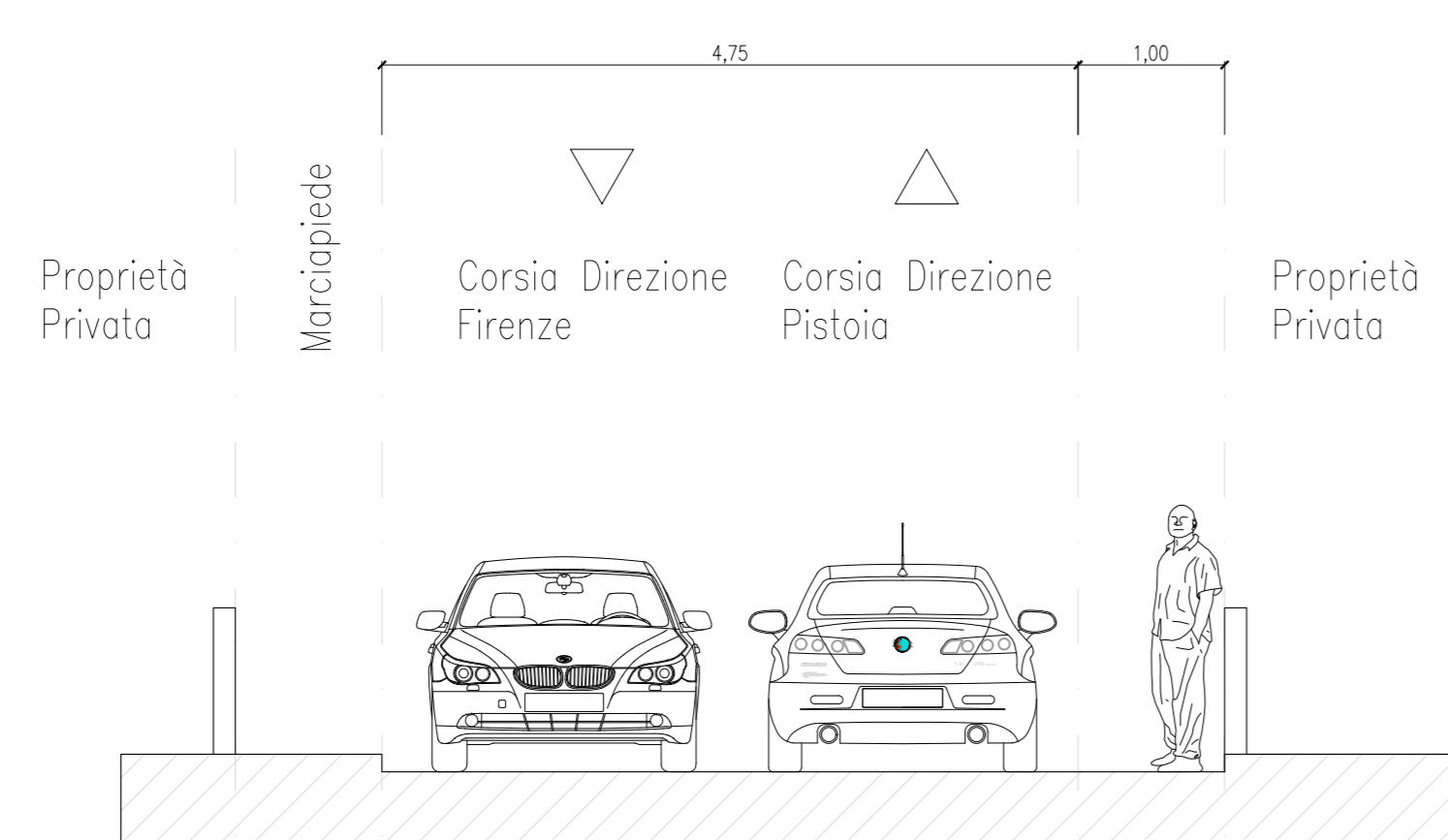
Stato Attuale via Aiaccia intersezione Via Mastrigalla scala 1:50
