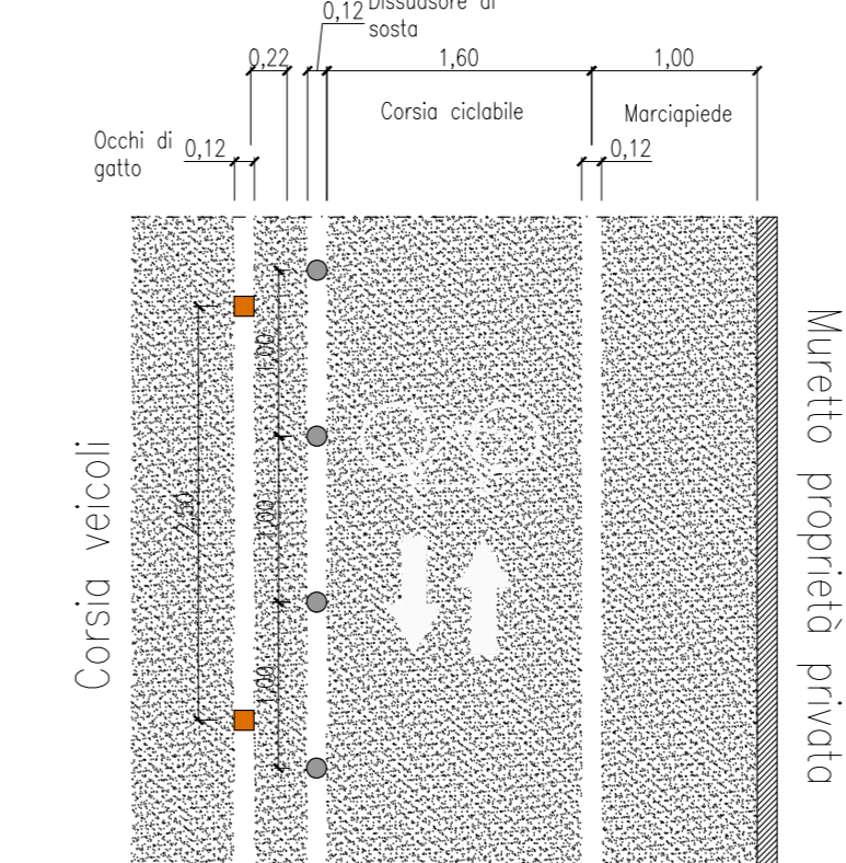
Particolare sistemazione in pianta scala 1:50
