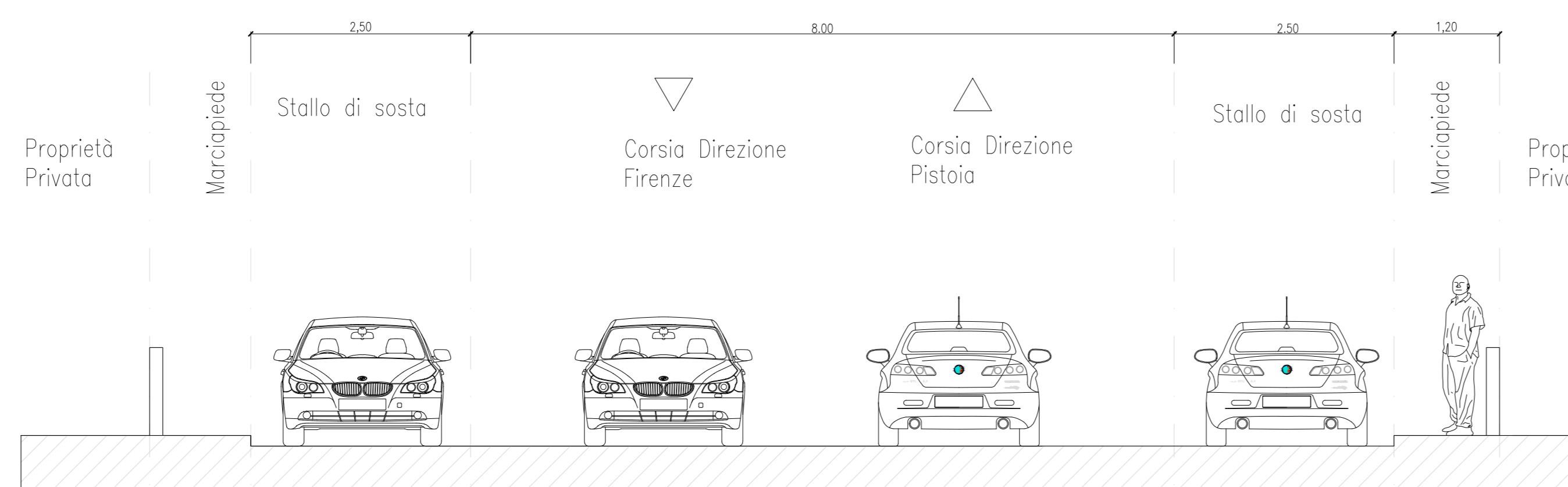
Stato Attuale via Cegoli, da via Monticello a via Dell'Amicizia scala 1:50
