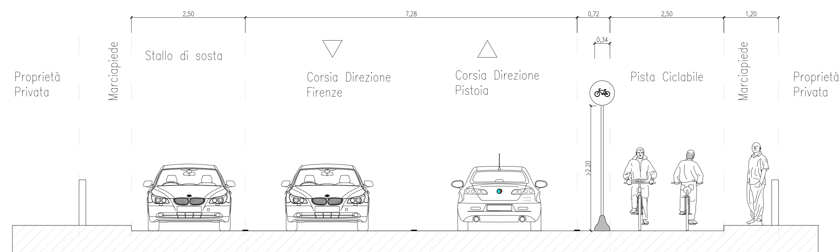
Stato Progetto via Cegoli, da via Monticello a via Dell'Amicizia scala 1:50
