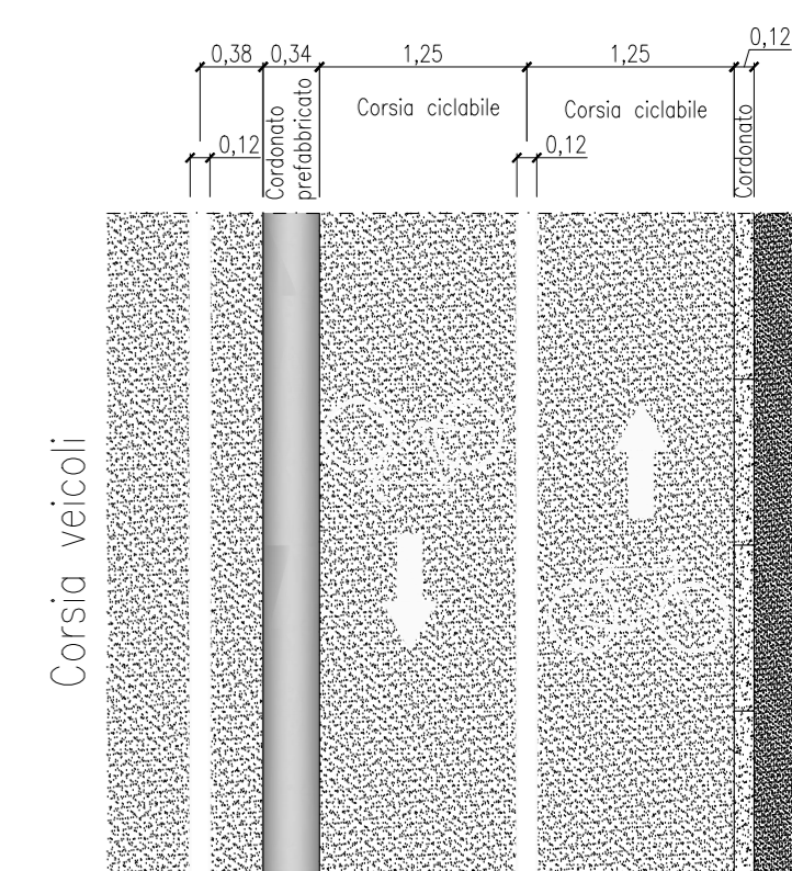
Particolare sistemazione in pianta scala 1:50
