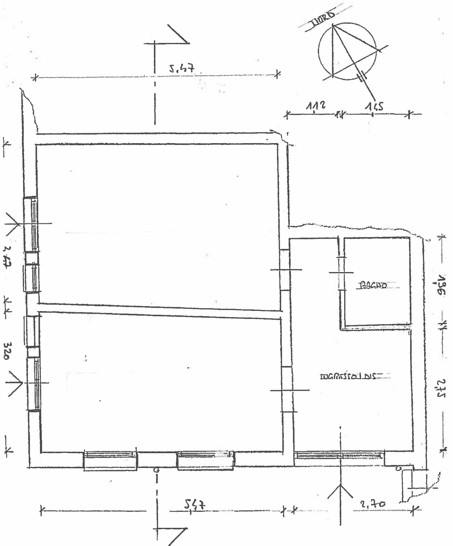
PIANTA PIANO TERRA - SCALA 1:50
