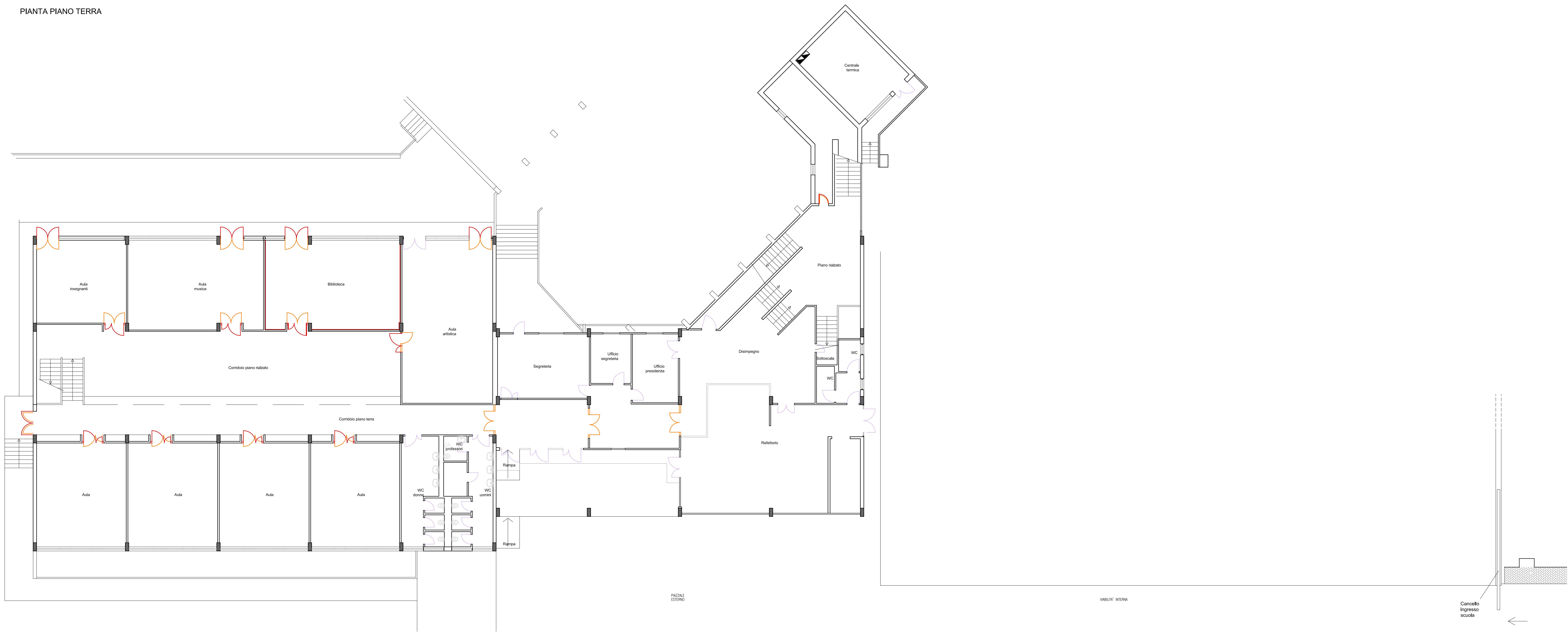
PIANTA PIANO PRIMO
