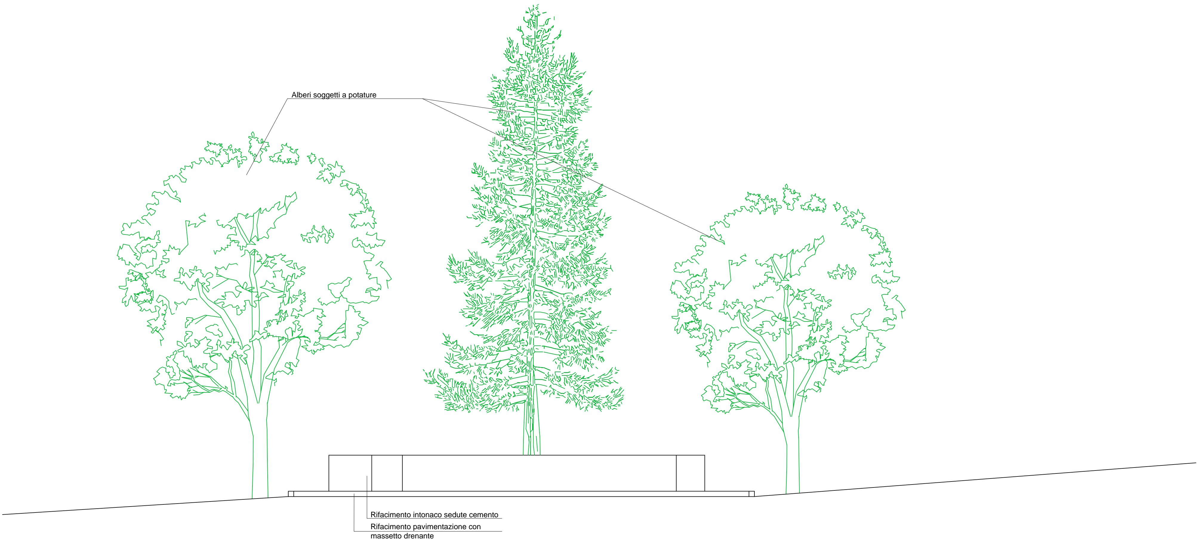
SEZIONE B-B' - STATO DI PROGETTO scala 1:50
