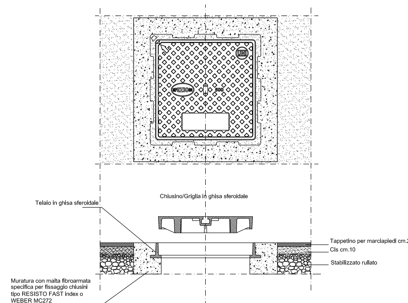
Particolare costruttivo ripristino in quota chiusini 1:10
