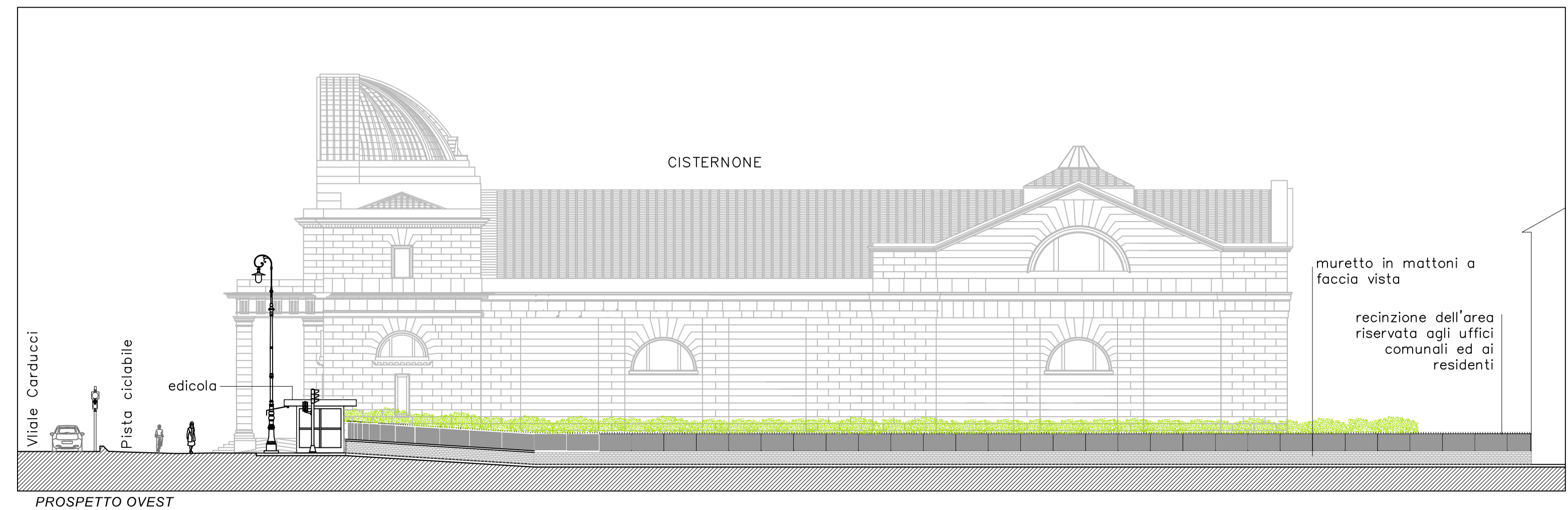
PROSPETTO OVEST
