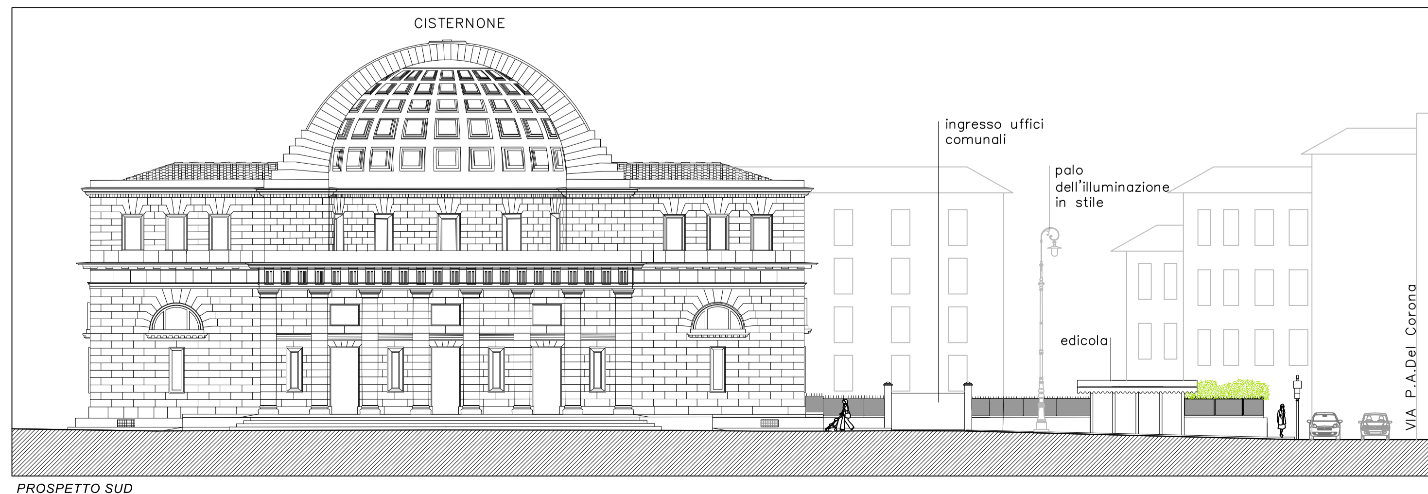
PROSPETTO SUD
