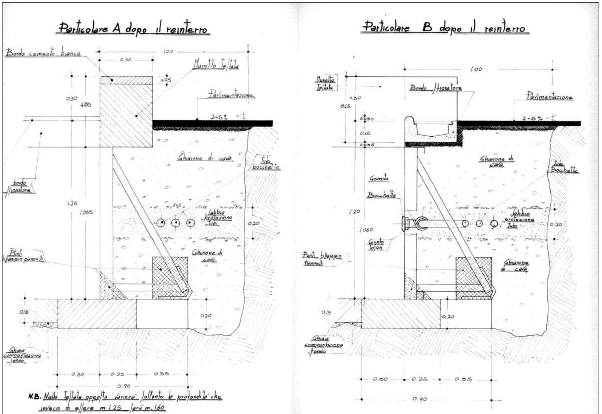
VASCA GRANDE - SEZIONI DI PROGETTO (1975) (NON IN SCALA)
