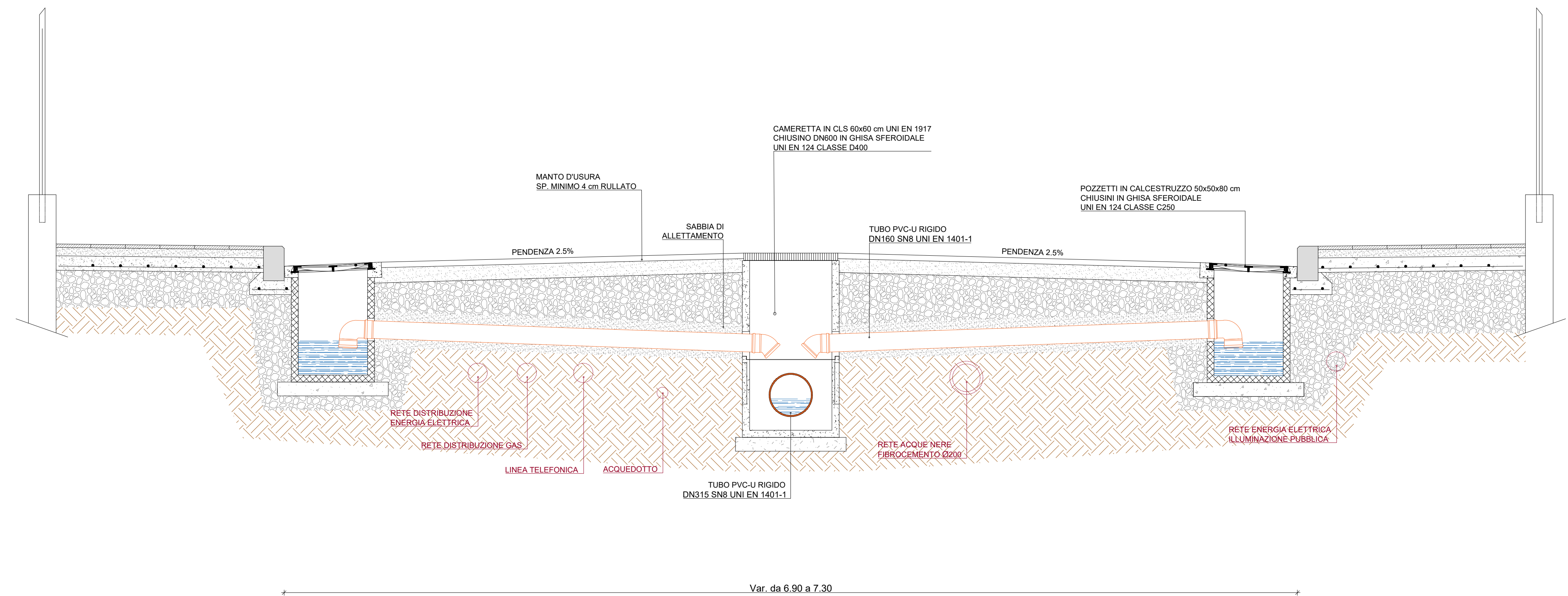
SEZIONE TIPO 1:20
